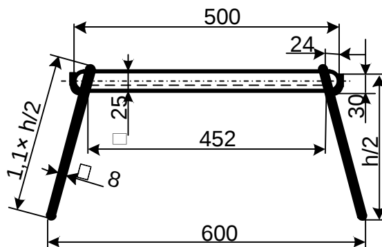
Рисунок 5.7 – Загальний вигляд та схема перерізу закладного елементу шва стискання, влаштованого за технологією розстановки закладних елементів (розміри показані в мм)
