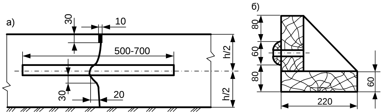
Рисунок 5.9 – Конструкція робочого шва (а) та шаблона-кутника для плити товщиною 220 мм
