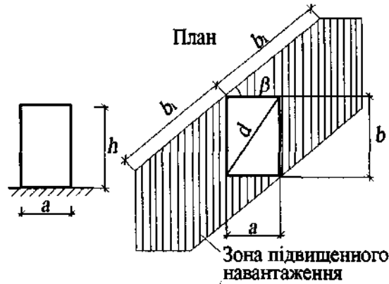
Схема 11. Ділянки покриттів, що примикають до вентиляційних шахт, які вивисшуються над покрівлю, та інші надбудови
