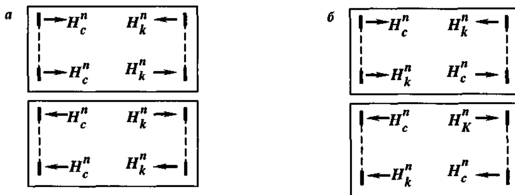
Рисунок 7.1. Варіанти прикладення бічних сил для чотириколісних кранів
