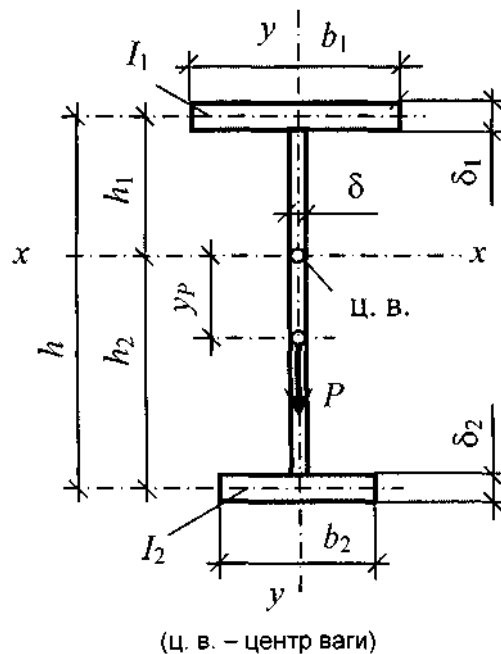
Рисунок Г.1 - Поперечний переріз балки з однією віссю симетрії і розвинутим верхнім поясом
