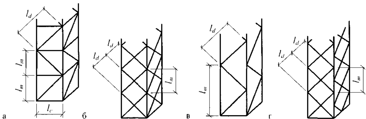
а - схема з вузлами, що збігаються в суміжних гранях (трикутні грати з розпирками); б - те саме (перехресні грати); в - схема з вузлами, що не збігаються в суміжних гранях (трикутні грати); г - те саме (перехресні грати)
