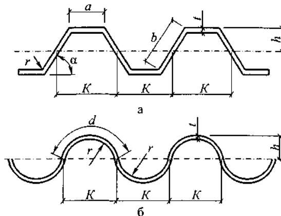
Рисунок 11.3 - Розрахункова схема стиснутого гофрованого листа
