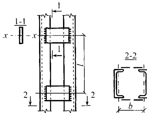
Рисунок 8.2 - Складений стрижень на планках
